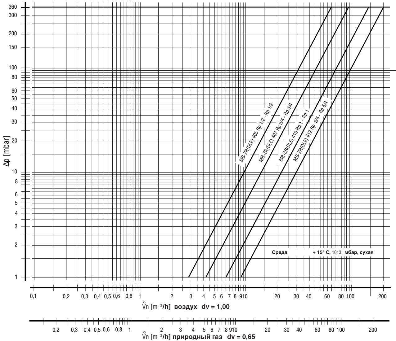
Диаграмма расхода 2 открыт механическим способом/ с микрофильмом / для выбора узла MB- использовать диаграмму расхода 1
